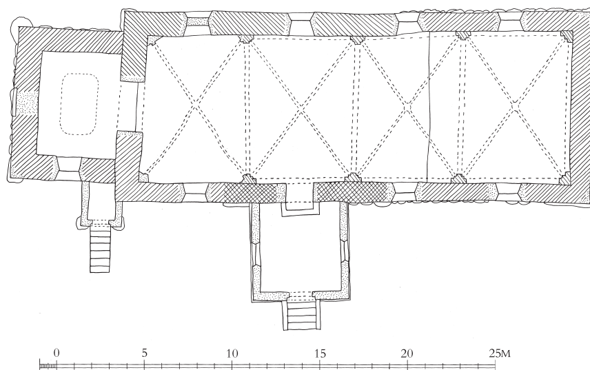
Fig. 9. Grundplan. 1:300. Målt af Ejnar Mindedal 1962, suppleret og tegnet af Pia K. Lindholt 2025. Signaturforklaring s. 9. – Plan. Key on p. 17.
