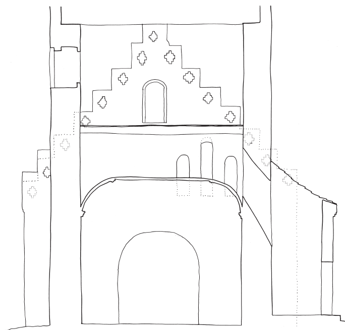
Fig. 13. Opmåling af det udvidede skibs vestgavl set mod øst. 1:150. Målt og tegnet af Pia K. Lindholt 2025. – Scale drawing of the extended nave's west gable, looking east.
