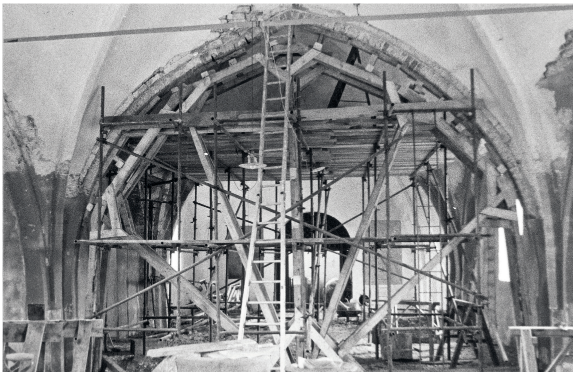
Fig. 25. Opretning af gjordbue ved den indre istandsættelse 1966-67 (s. 4574). Foto Anders Ploug-Sørensen 1966-67. I NM. – Resetting of a transverse rib at the interior refurbishing in 1966-67.
