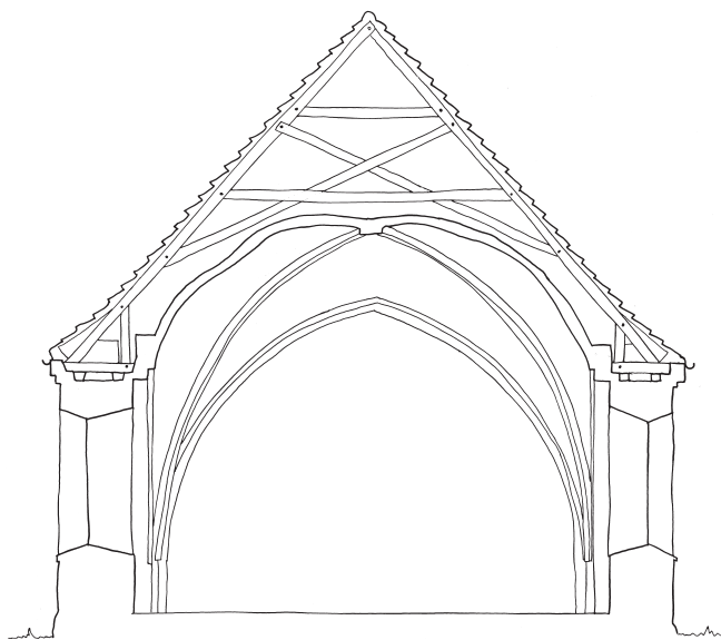
Fig. 8. Tværsnit. 1:150. Efter opmåling fra anden halvdel af 1800-tallet, suppleret og tegnet af Pia K. Lindholt 2025. – Cross-section.
