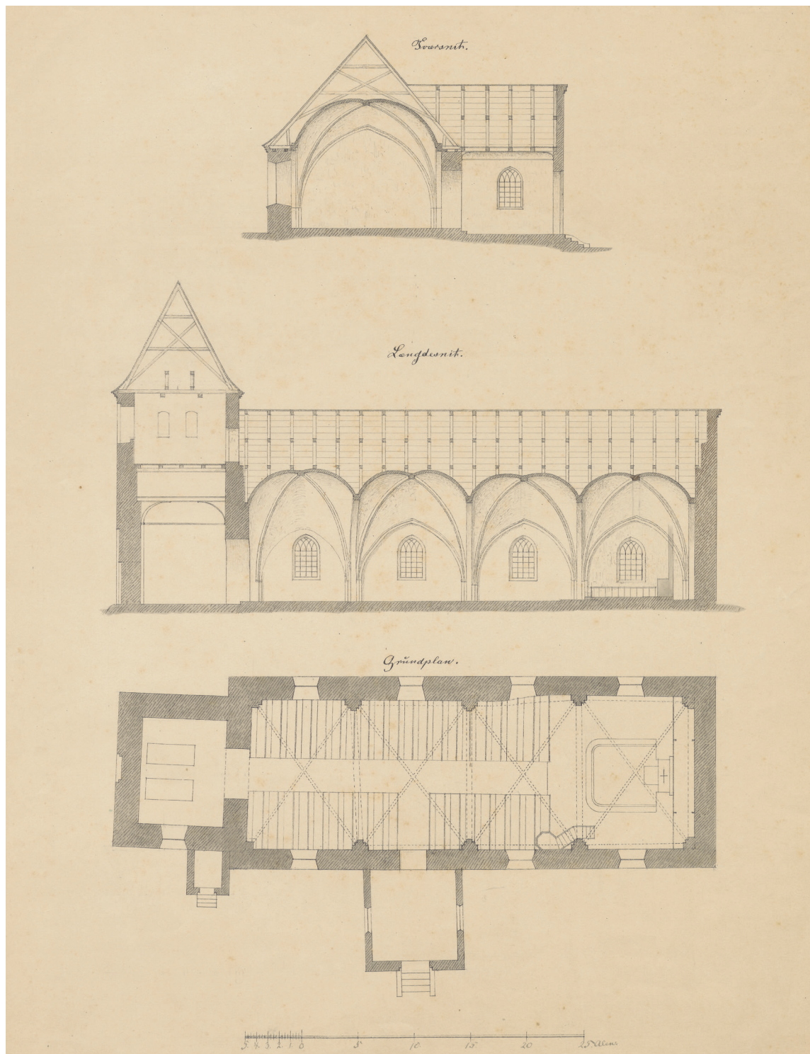
Fig. 20a-c. Opmåling af kirken, anden halvdel af 1800-tallet. 1:300. a. Tværsnit set mod øst. b. Længdesnit set mod nord. c. Grundplan. I KB. Kunstbiblioteket. – Scale drawing of the church, second half of the 1800s. a. Cross-section looking east. b. Longitudinal section looking north. c. Ground plan.
